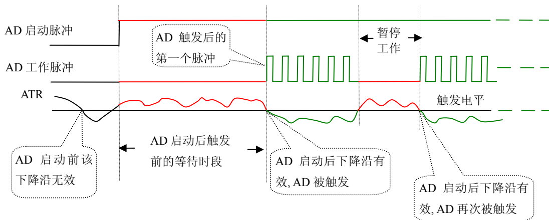
图 6.4 低电平触发
