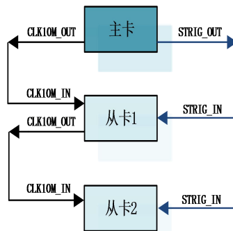
图4-10-1 主从卡级联
