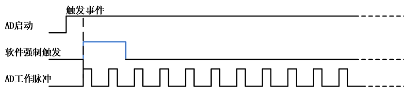
图 4-8-3 AD 软件触发
