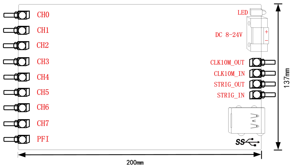
图 3-2-1 USB8584\8582 板卡尺寸图
