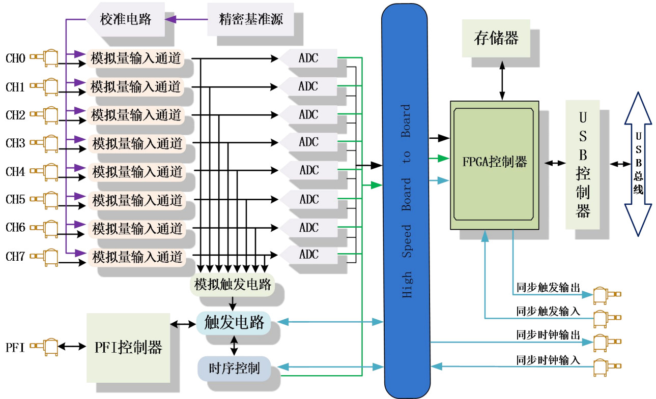
图 3-1-1 USB8584\8582 系统框图
