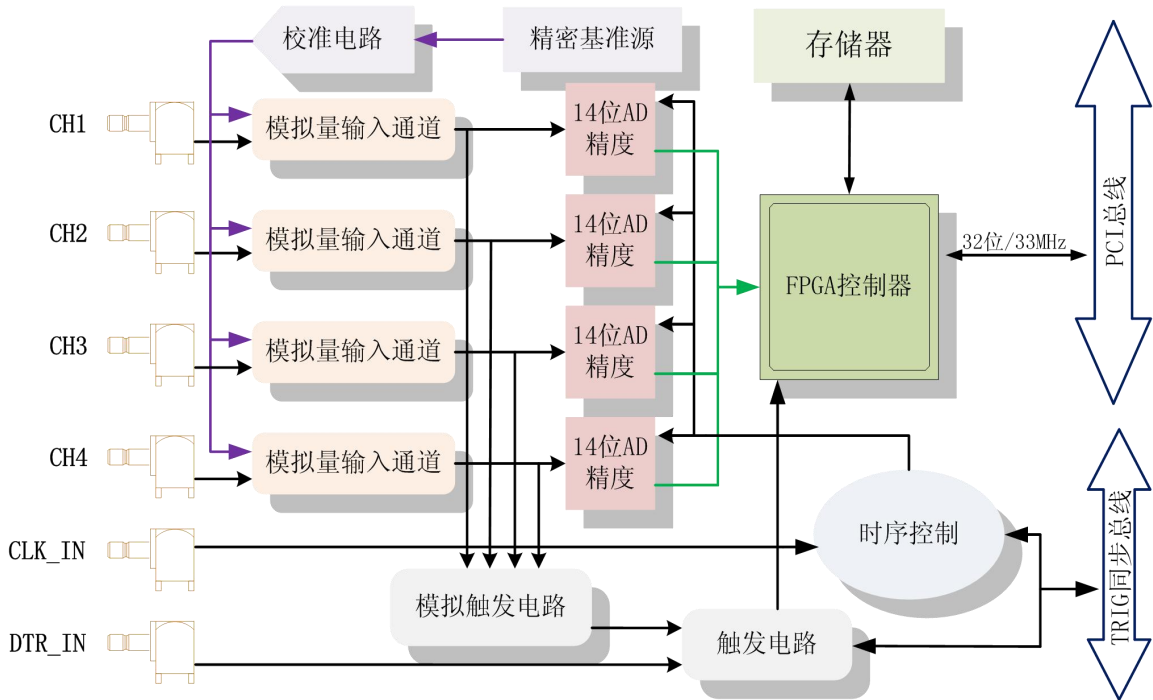
图 3-1-1 PCI-8514B/8504B 系统框图
