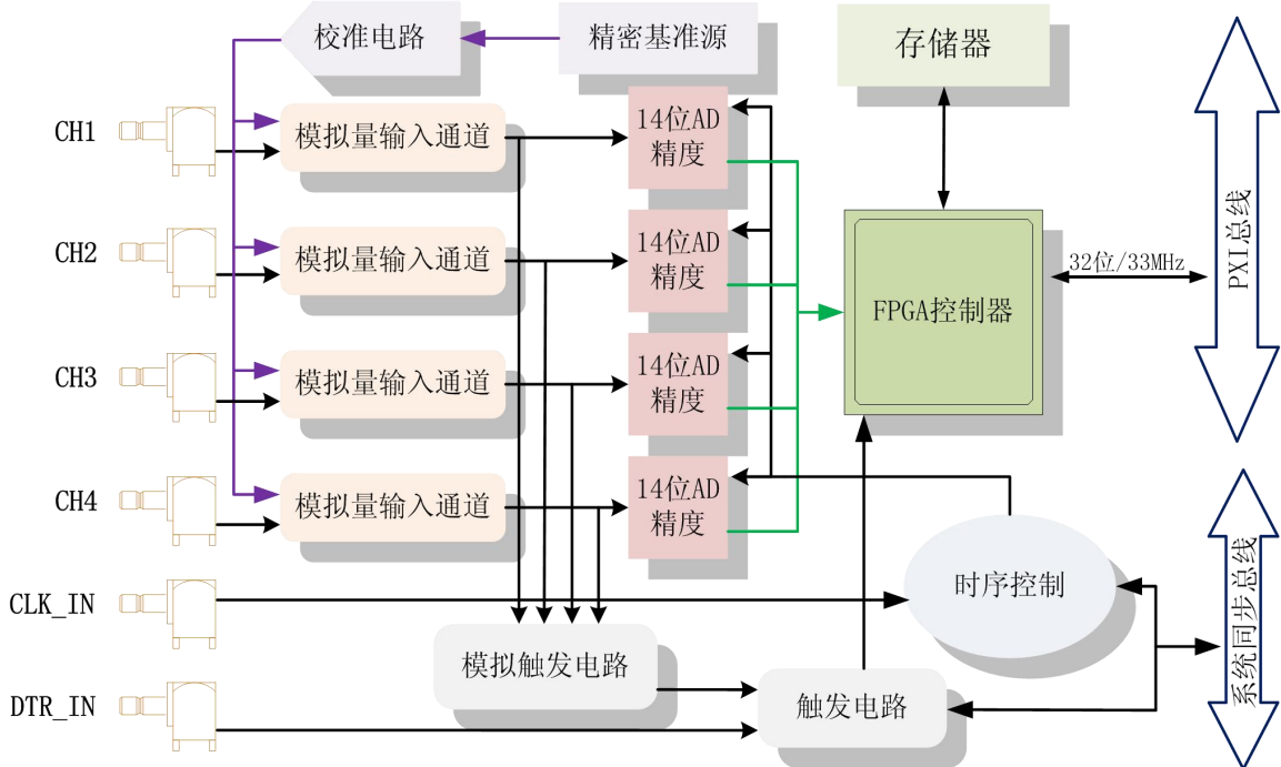
图 3-1-2 PXI-8514B/8504B 系统框图
