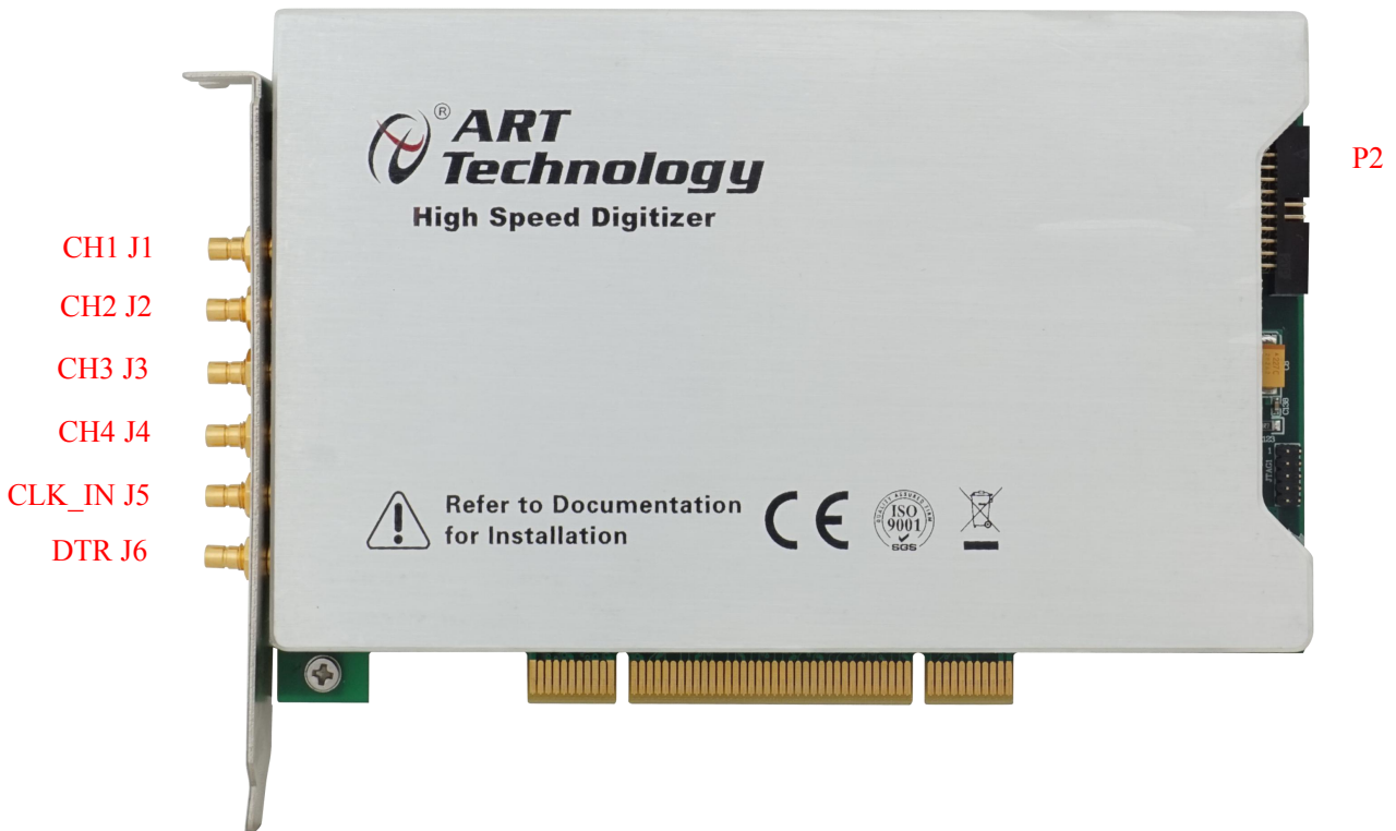
图 3-3-1 PCI8514B/8504B 元件布局图
