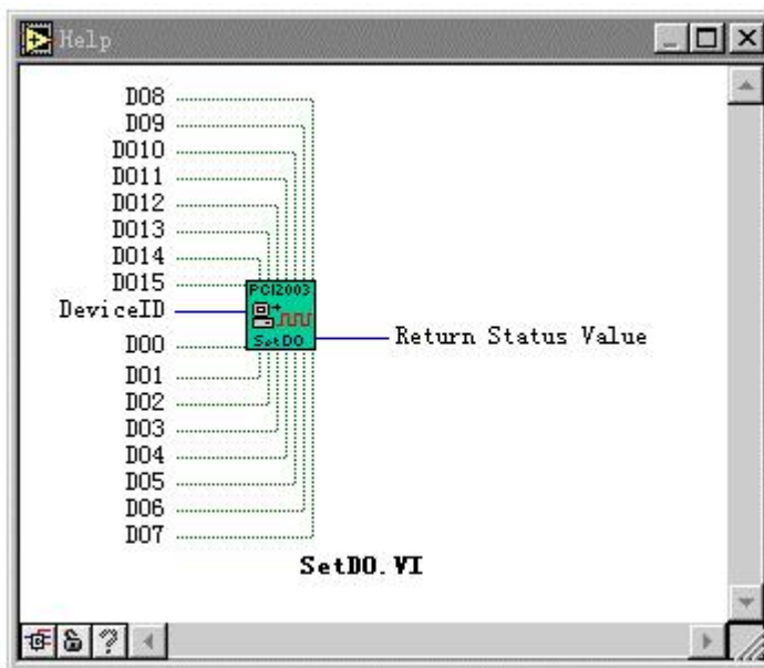
图 12 开关量输出驱动器
